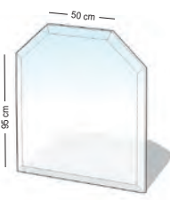
Glasbodenplatte glasklar, mit geschliffenen Kanten Stärke 6 mm Fase 20 mm
