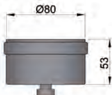
Kondenskapsel
