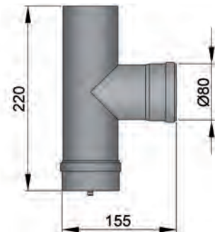
T-Stück mit Kondenskapsel
