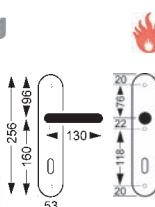
Schutzbeschlag Mod. IKARUS mit Kernziehschutz
