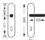
Schutzbeschlag Mod. HEROLD mit Stahleinlage im Außenschild
