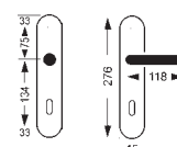
Schutzbeschlag Mod. ALT WIEN mit gehärteter Stahleinlage
