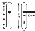
Schutzbeschlag Mod. HEROLD mit Stahleinlage im Außenschild
