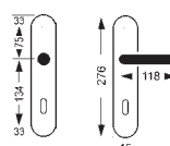
Schutzbeschlag Mod. ALT WIEN mit gehärteter Stahleinlage
